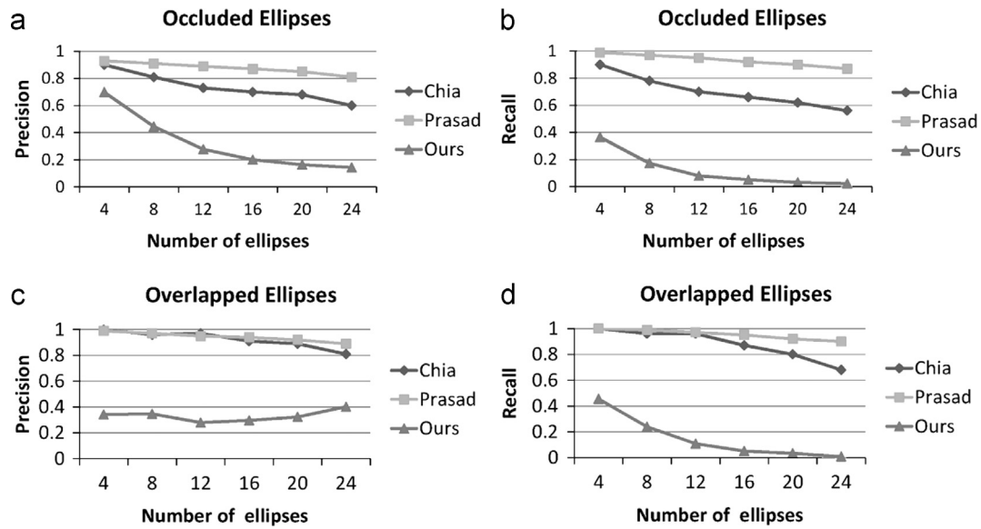
Fig. 17. Evaluation on Dataset Chia [24]. (a) Precision. (b) Recall. (c) Precision. (d) Recall.
